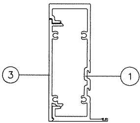
JAMB 'J1'
