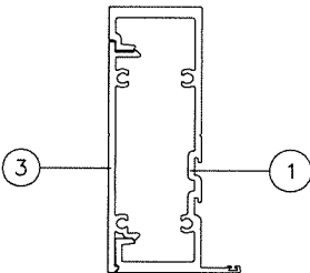
JAMB 'J1'
