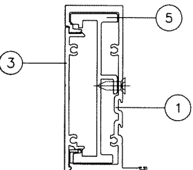
JAMB 'J2'
